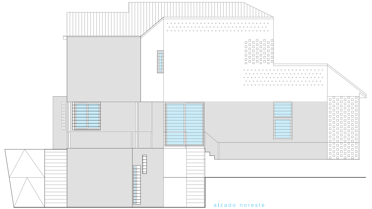
alzado noreste
