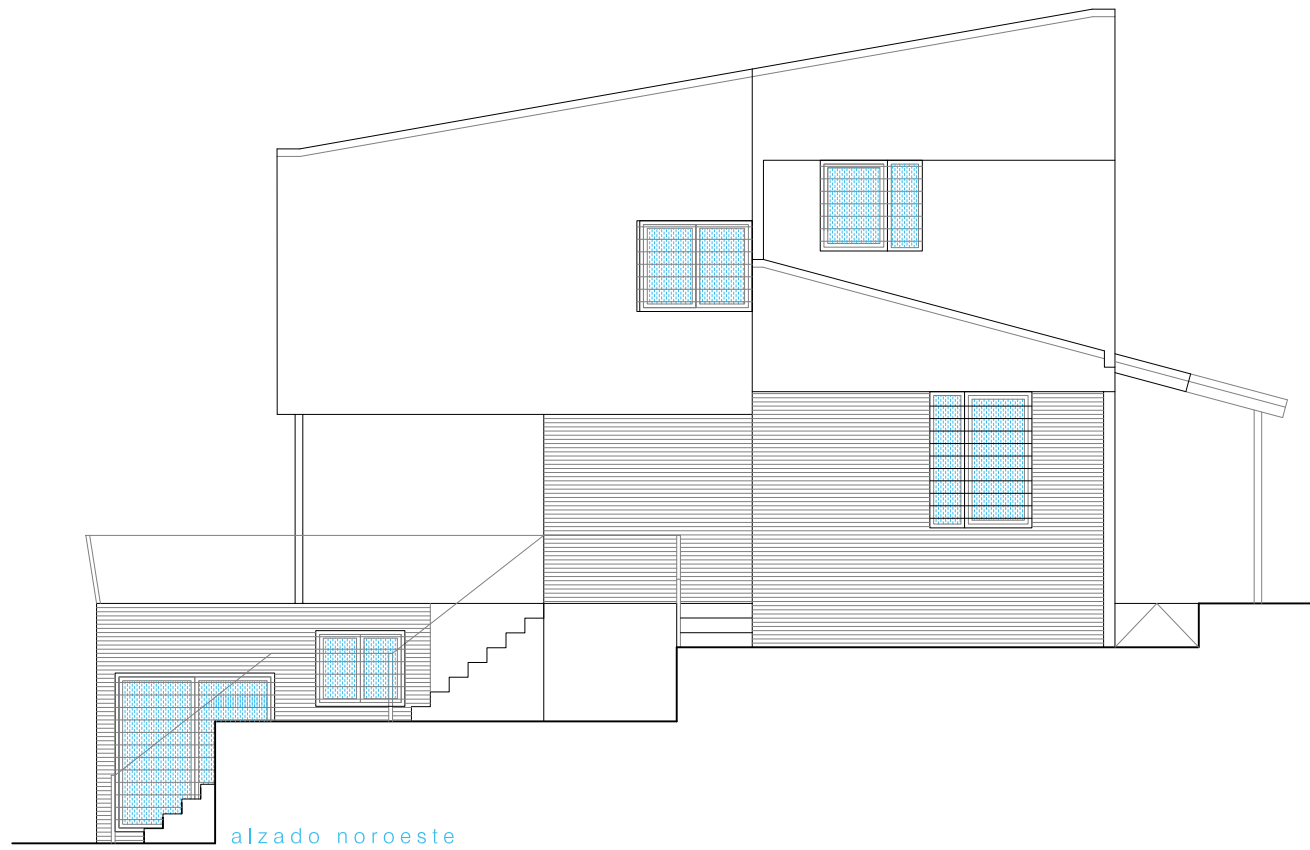
alzado noroeste
