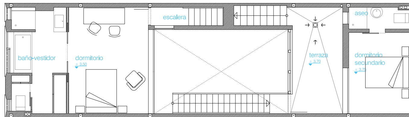
planta primera
