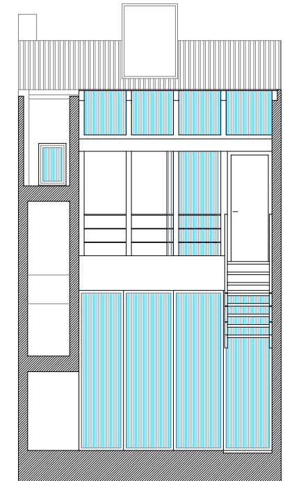
fachada-sección patio CC' (sur)
