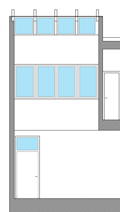
fachada-sección patio BB' (norte)
