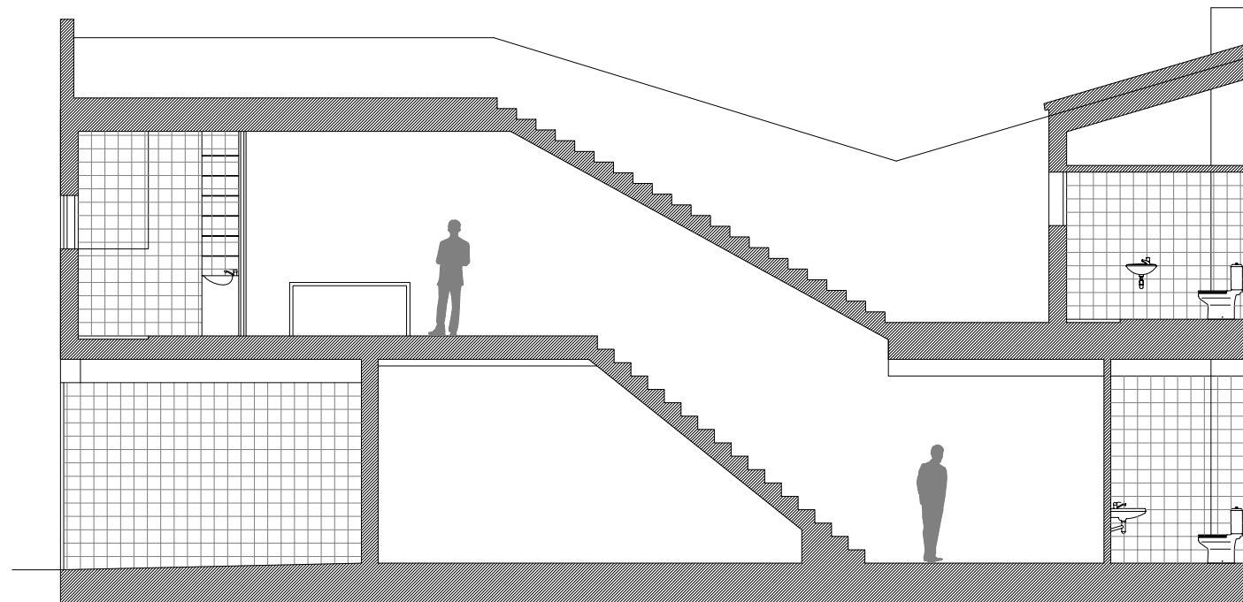
sección DD'
