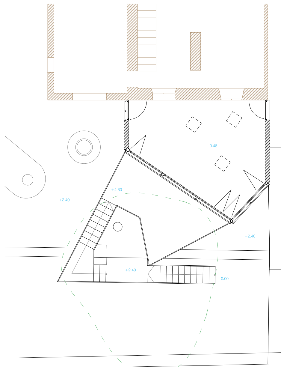
planta primera
