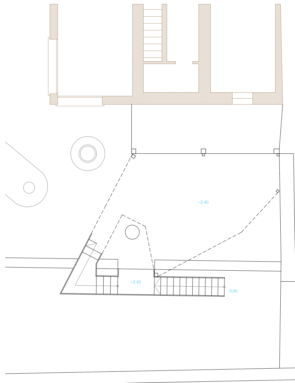
planta baja
