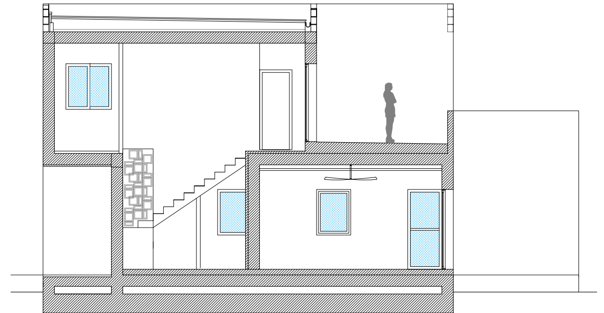
sección A-A'
