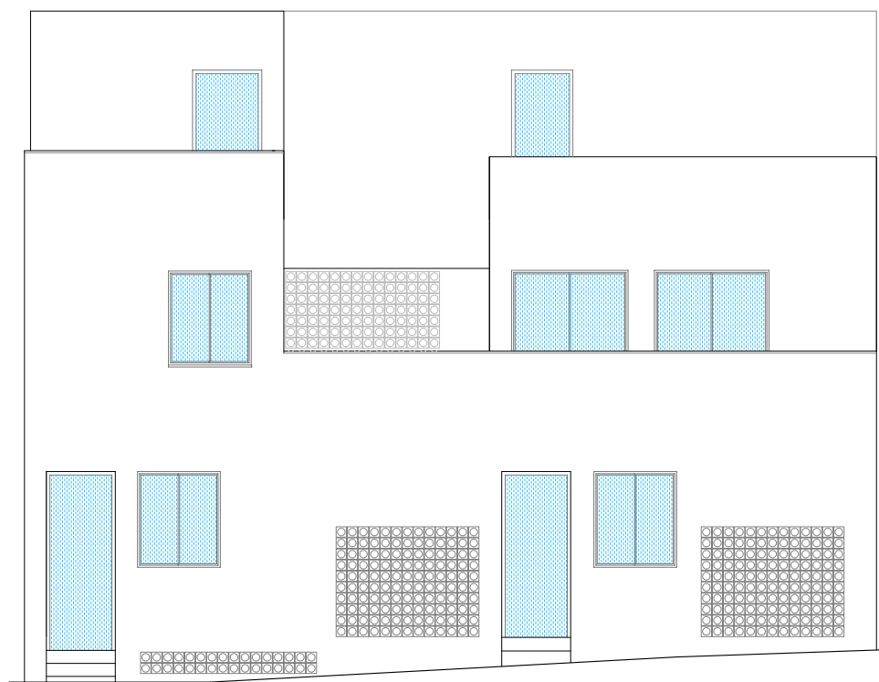
alzado norte
